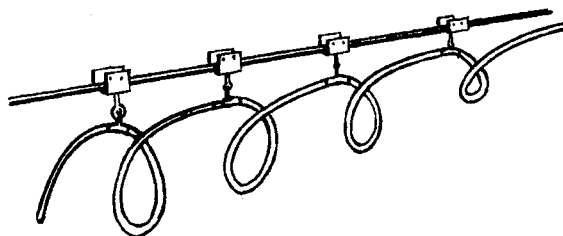
(d) Festooned Round Cable
