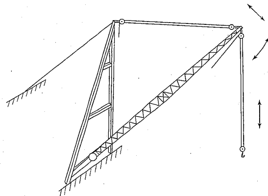
Fig. 6-0.2.1-1 A-Frame Derrick
