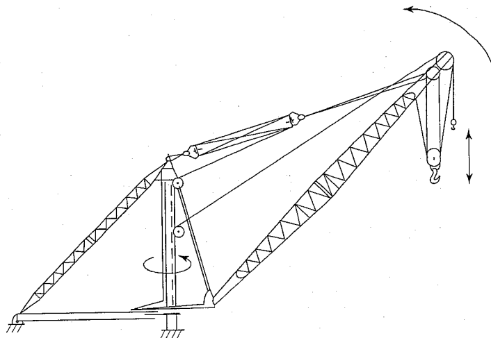
Fig. 6-0.2.1-8 Stiffleg Derrick
