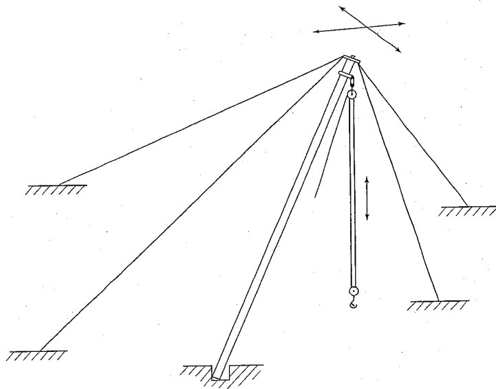
Fig. 6-0.2.1-5 Gin Pole Derrick
