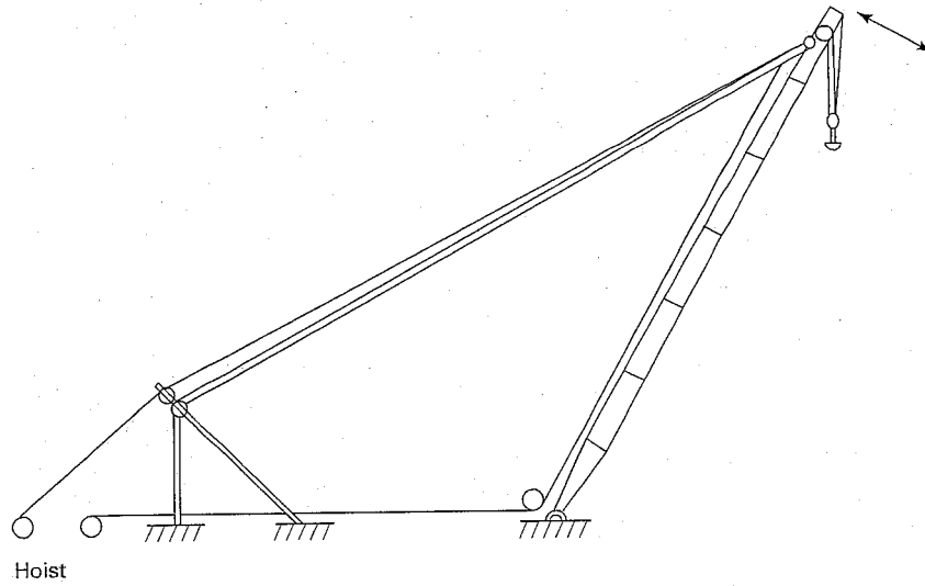
Fig. 6-0.2.1-7 Shearleg Derrick
